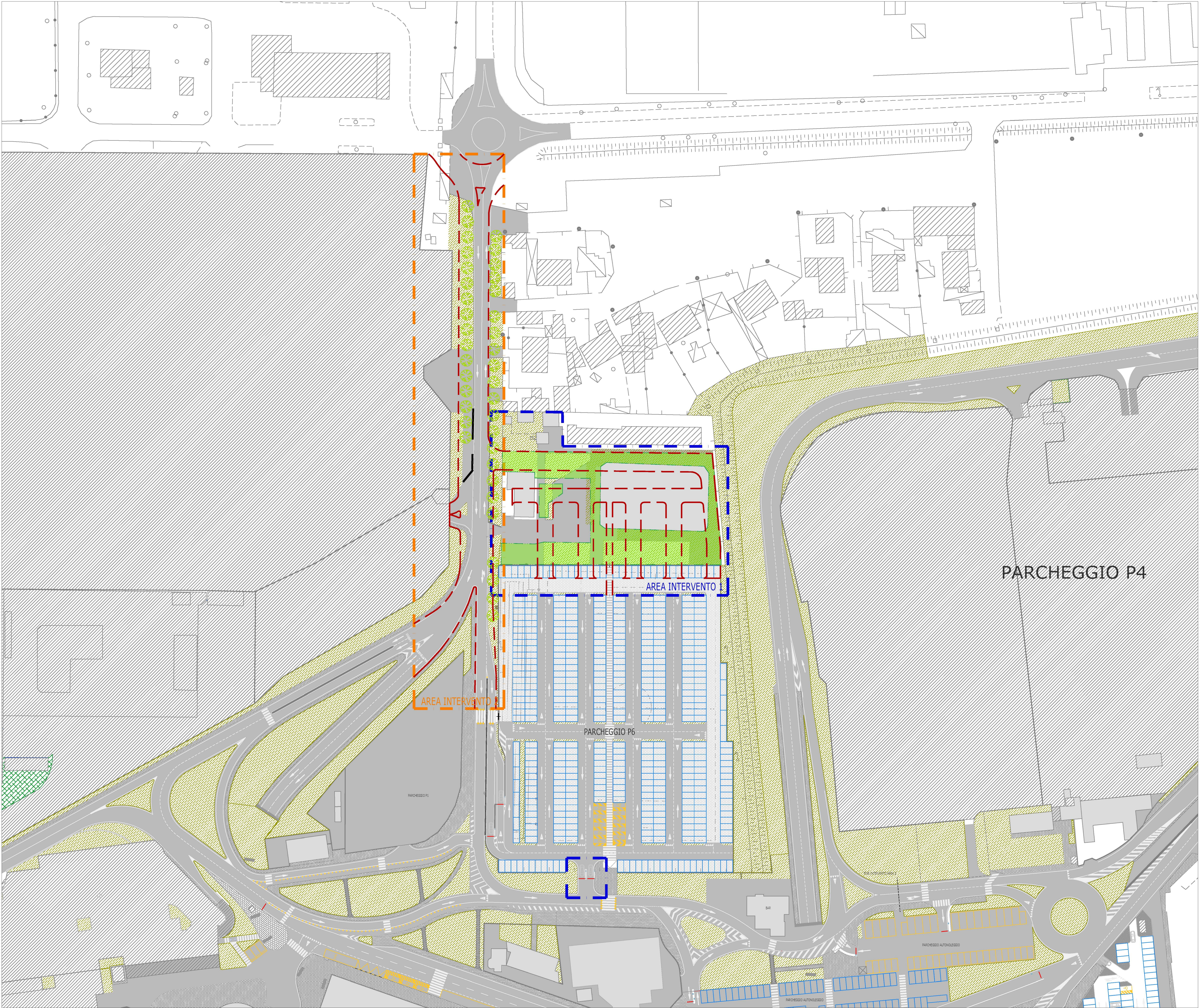
Planimetria generale con individuazione aree di intervento Scala 1:500
